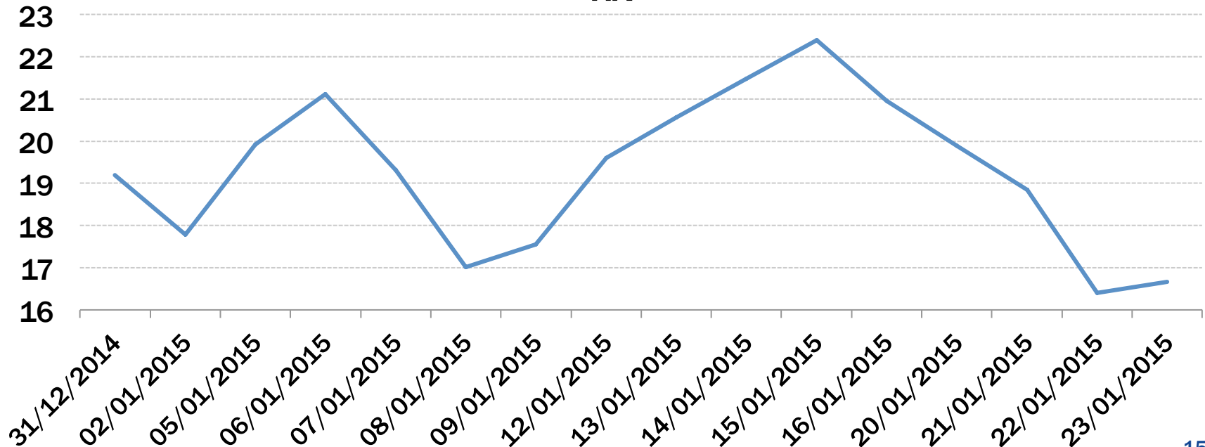
VIX
